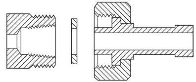
CGA 705 1.125-14UNS-2A-RH-EXT
