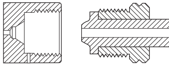
CGA 703 1.125-14NGO-LH-INT
