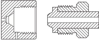
CGA 702 1.125-14NGO-RH-INT
