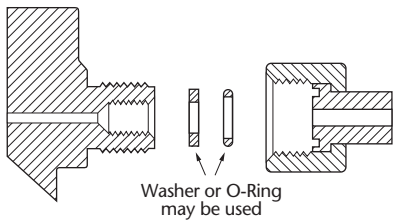
CGA 180 .625-18UNF-2A-RH-EXT
